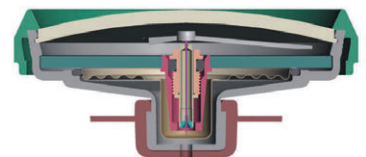
DuraShock Messwerk
